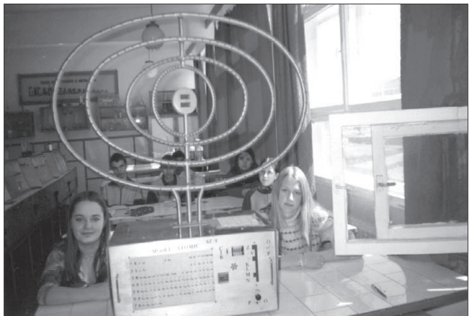
Elektronikus atommodell
